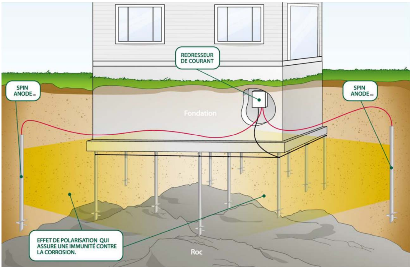
Figure 9 - Fonctionnement de la protection cathodique
