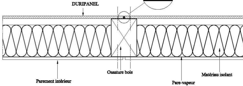
Détail A : Panneau de mur*
