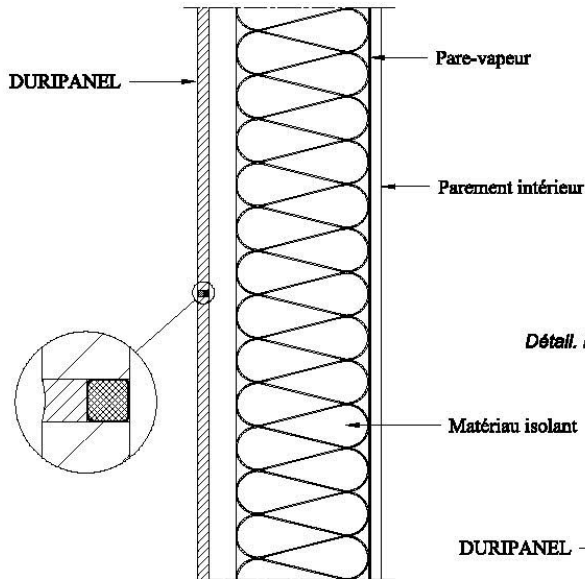
Détail. A: Panneau de mur*
