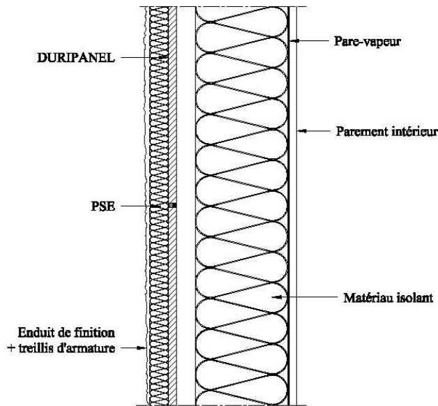
Détail. C: Panneau de mur avec finition par enduit sur isolant
