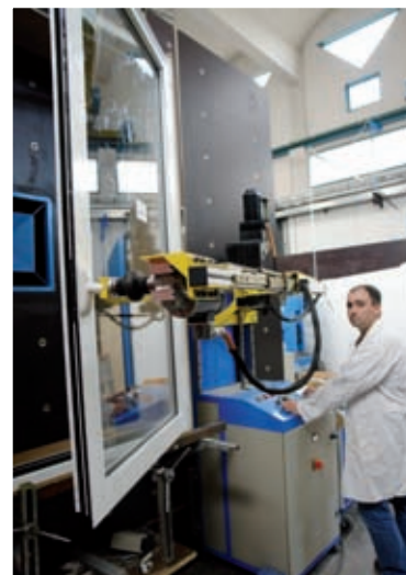
Essai d'endurance
